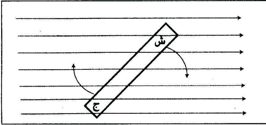
الشكل (38): تأثير حقل مغناطيسي متجانس على ثنائي قطب هو خلقي قوة فتل تجعله يدور بحيث يكون القطب الشمالي للمغناطيس مصطفا مع خطوط الحقل.
